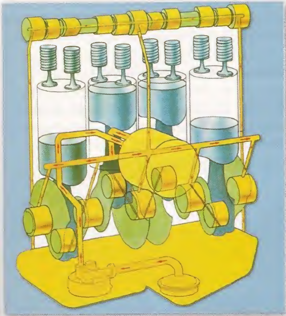
Circuito de lubricación
